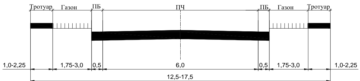
а) Поперечные профили распределительных (IVА-р, IVБ-р категории) и подъездных (IVА-п, IVБ-п категории) автомобильных дорог
